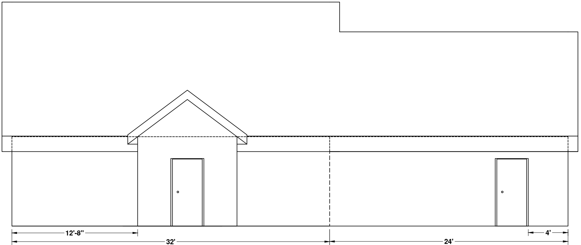
Right elevation 3
